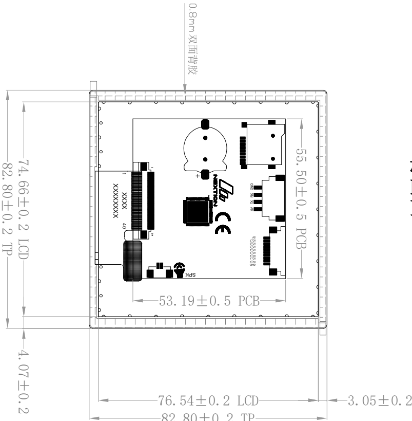
背面图
